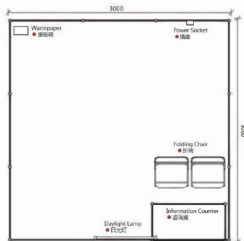
Layout Plan 平面图
